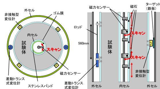
図2 変位計測システムのご概念
