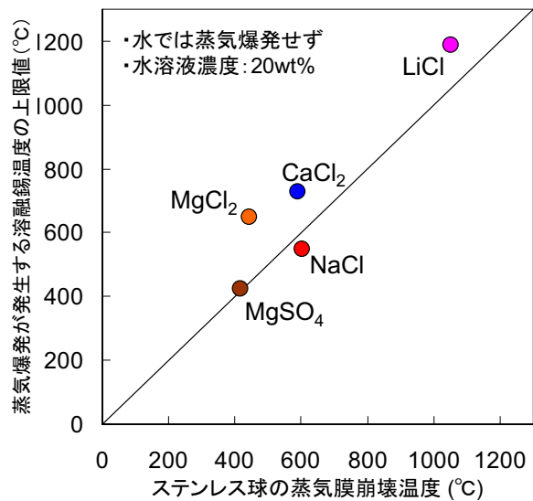
図 4 ステンレス球の蒸気膜崩壊温度と蒸気爆発が発生する溶融錫温度の相関
