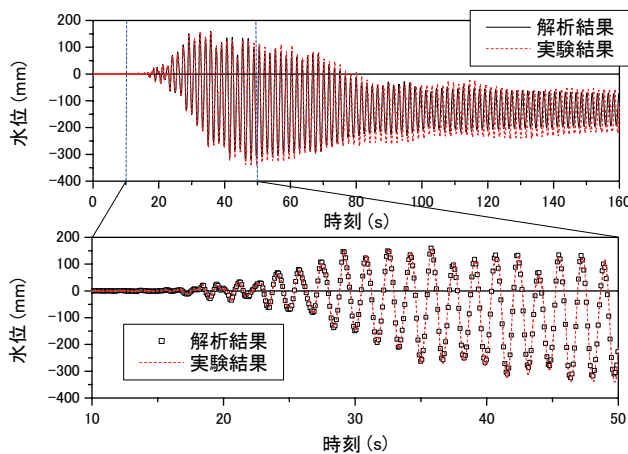
図4 水位の時刻歴応答の比較
