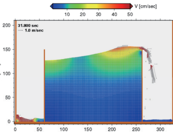
図3 スロッシング解析法の開発
