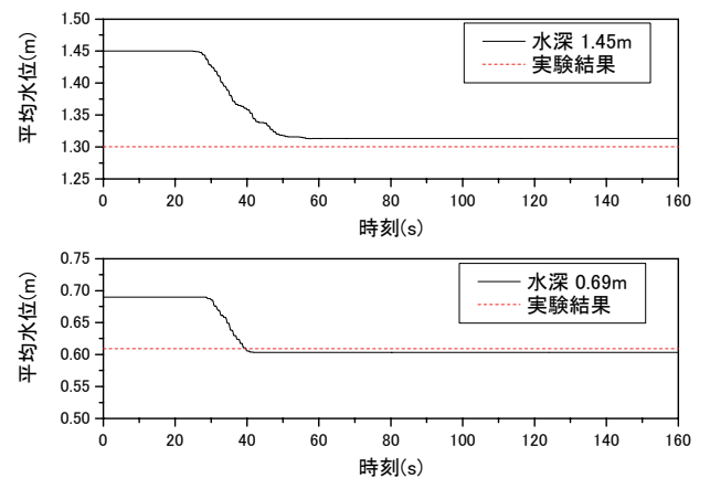
図5 平均水位の時刻歴応答の比較
