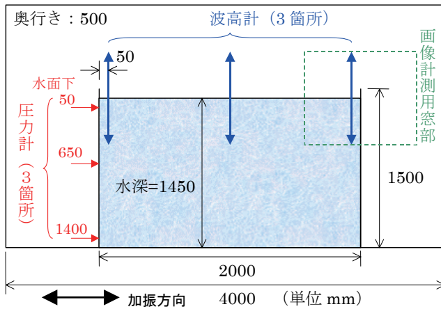
図1 タンク模型の形状とセンサー配置図
