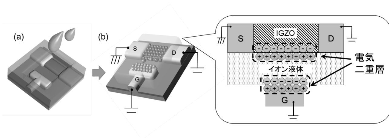
図2：IGZO 薄膜トランジスタにイオン液体が形成する電気二重層を用いた高性能化のイメージ図
