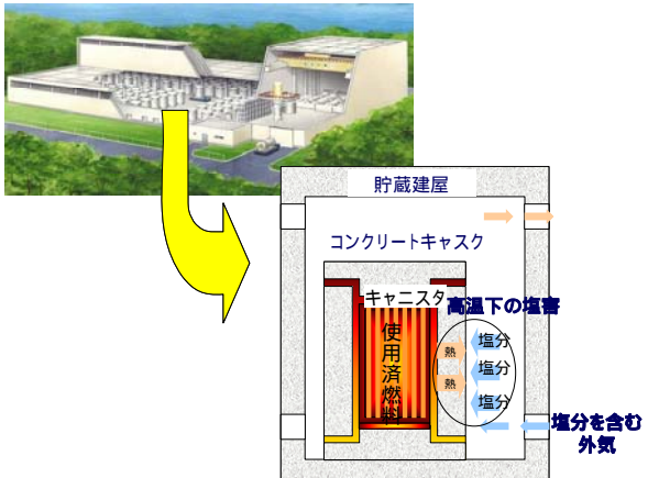
図1 沿岸立地の中間貯蔵施設に想定される塩害
