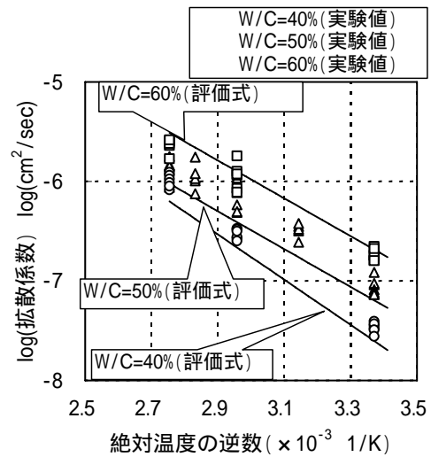
図2 コンクリート中の塩化物イオンの拡散係数
