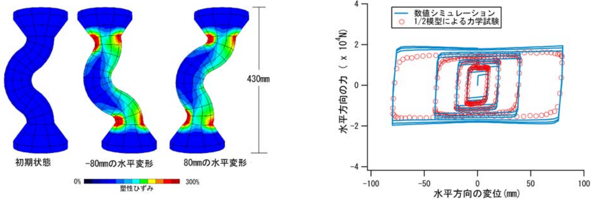
図1 鉛ダンパーの数値シミュレーションと力学試験
