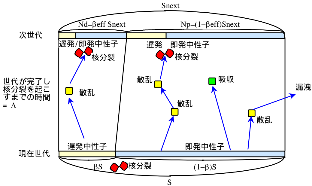
図1 開発した動特性パラメータ計算手法の概念。MCNPコードでは現在世代の中性子発生数 S と次世代の中性子発生数 S_{next} を用い実効増倍係数 k_{eff} を k_{eff} = S_{next} / S で評価している。原子炉運転中は S_{next} = S である。開発手法では遅発中性子の生み出す次世代中性子数 N_d を用いて k_{eff} = N_d / S_{next} で k_{eff} を評価する。またMCNPコードで計算される個々の中性子の寿命を、その中性子が生み出す次世代中性子数で重み付けして平均化することで k_{eff} を得る。
