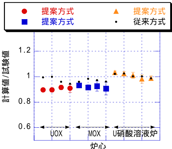
図3 本手法による k_{eff} / S の計算精度と従来法による計算精度の比較
