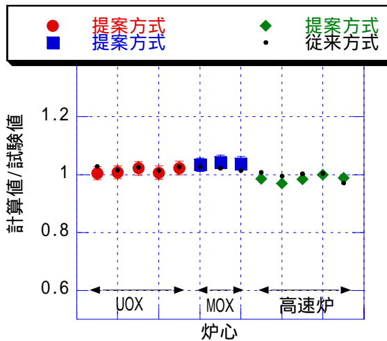
図2 本手法による k_{eff} の計算精度と従来法による計算精度の比較
