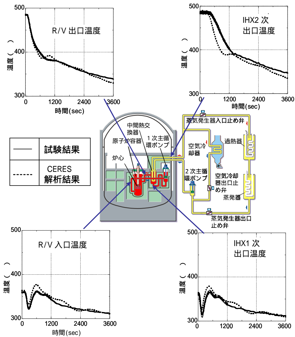
図1 もんじゅ冷却系の過渡温度変化とCERESコードによる解析結果の比較
