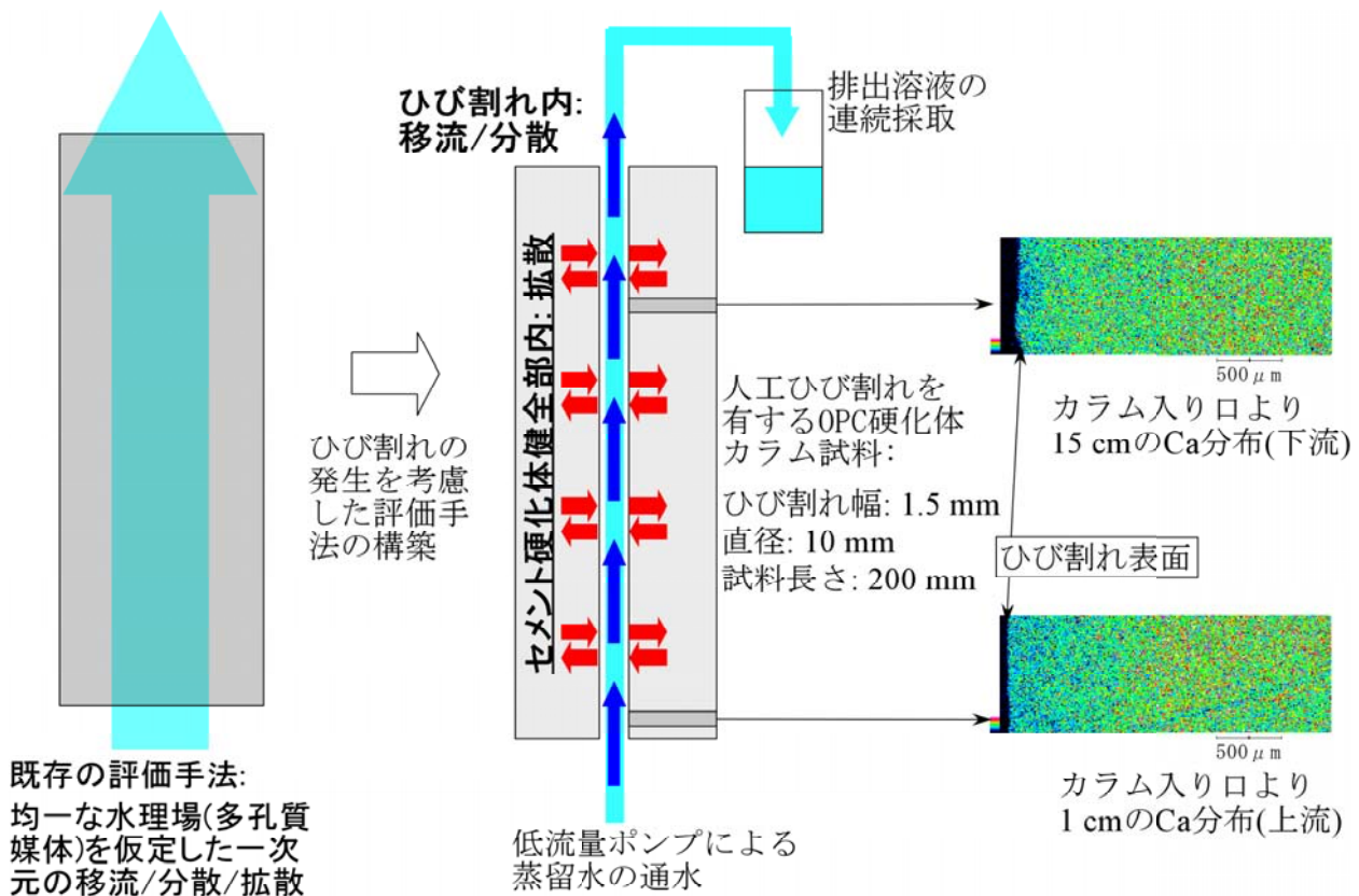
図2 単一人工ひび割れセメント硬化体の評価体系(実験、モデル化)と固相中の組成変化観察結果 ひび割れを有するセメント系材料内部の不均一な水理場を、ひび割れに平行な方向のひび割れ内の移流とひび割れに垂直な方向のマトリクス拡散の組み合わせで表現した物質移行モデルを構築し、解析コードのプロトタイプを開発した。単一ひび割れを模擬した実験により、変質挙動の定量的データを取得した。固相については、カルシウム成分の溶脱により、ひび割れ表面から内部に向かって生じた組成の分布を観察した。
