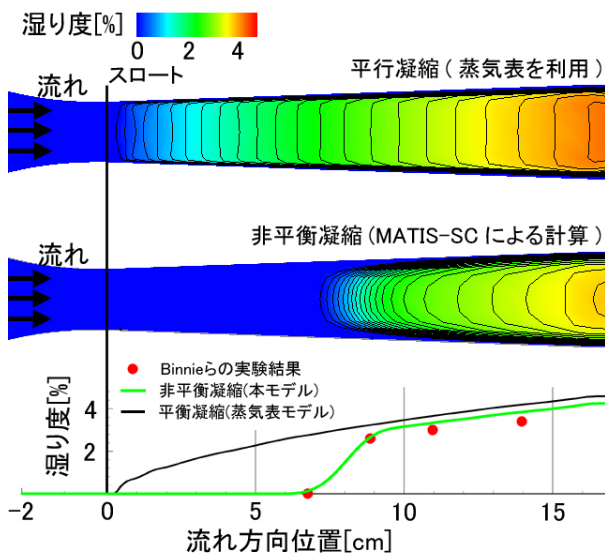
図 3 超音速ノズル内の湿度の可視化図(上・中図)と流れ方向の湿度分布(下図) (流入圧力 65.5kPa, 流入温度 400.15K) MATIS-SC の結果は、ノズル内での急激な湿度の変化(非平衡凝縮)が発生しており、実現象である実験と良い一致を見ている。蒸気表を利用した計算では湿度が徐々に変化しており、実験と合わず実現象を捉えられていない。
