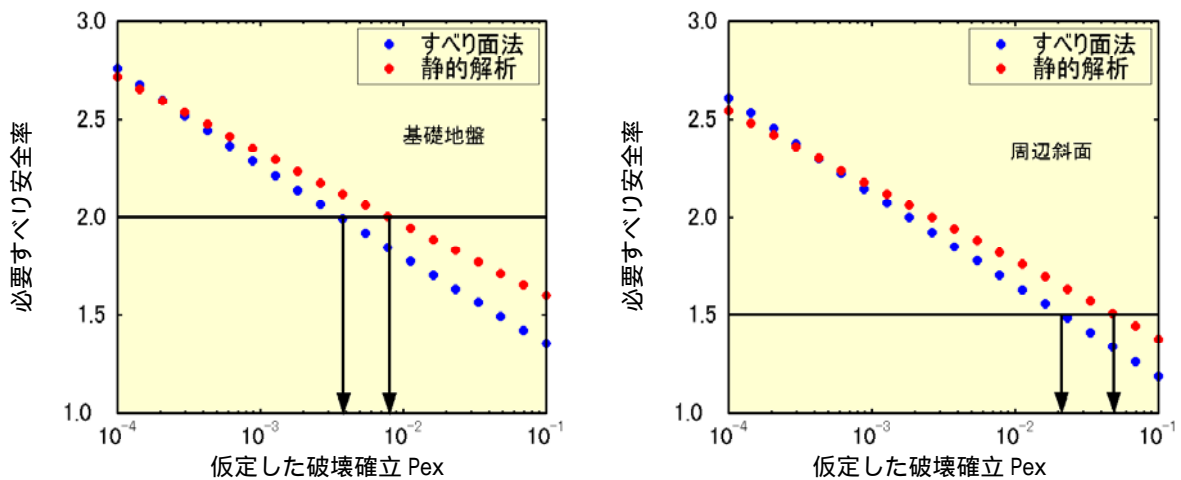
図3 必要すべり安全率
