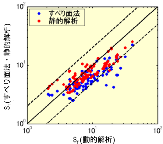
図1 既設の原子力発電所の基礎地盤及び周辺斜面の調査結果(同一の構造物に対してすべり安全率を評価した結果は、動的解析 > 静的解析 > すべり面法の順になる傾向がある。)
