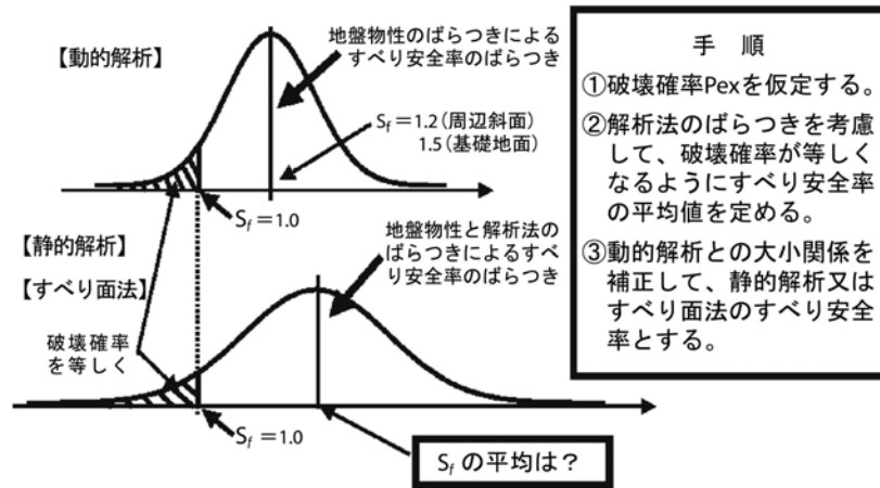
図2 検討方法の概要
