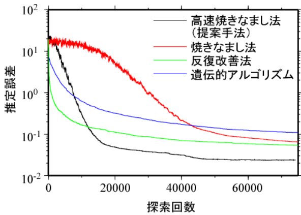
図1 各種手法による解探索能力の比較
