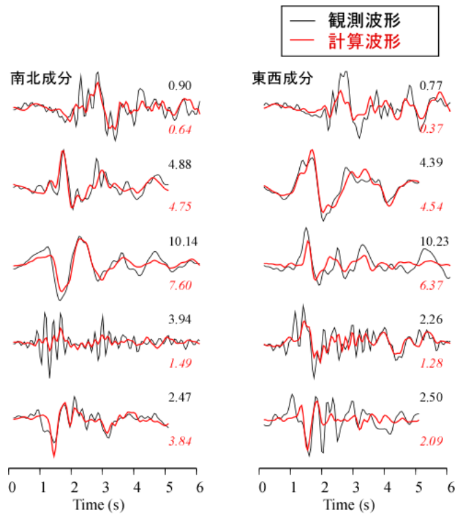
図3 観測波形と解析結果に基づく計算波形の比較
