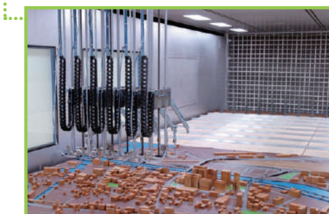
乱流輸送モデリング風洞
