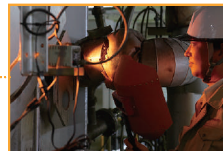
石炭燃焼特性実証試験装置
