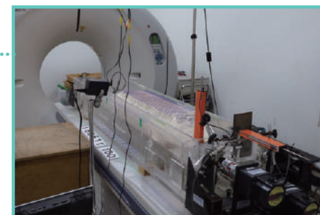
ヘリカルCT線装置
