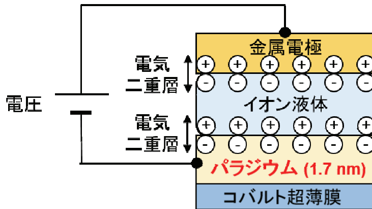
図1: 実験に用いた素子の模式図
